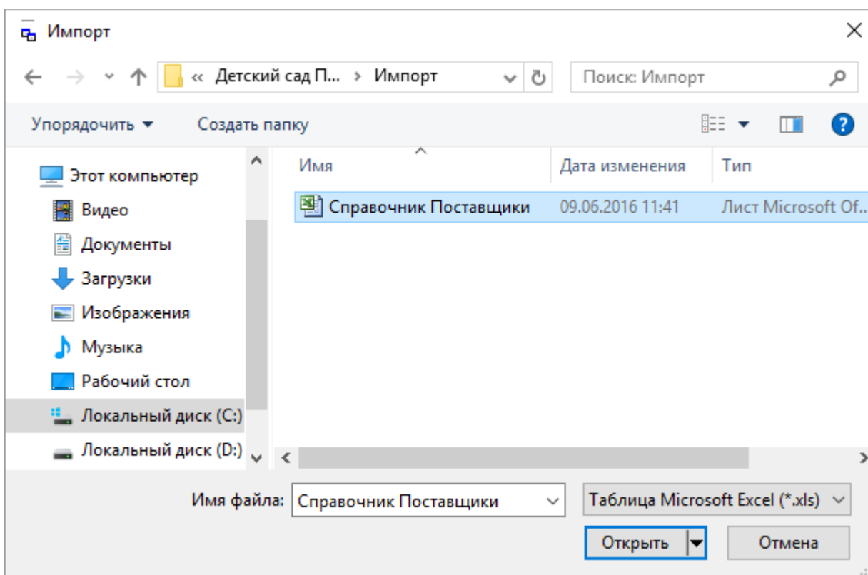
Окно «Импорт»
