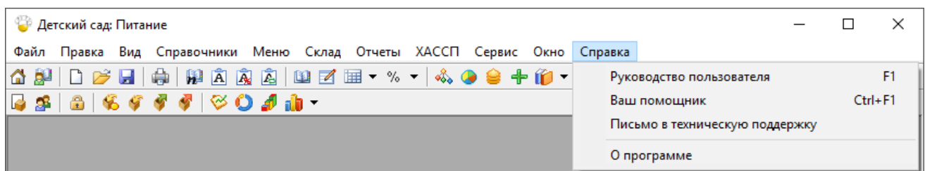
Меню «Справка»
