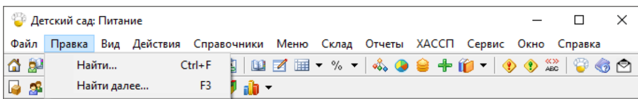
Меню «Правка»
