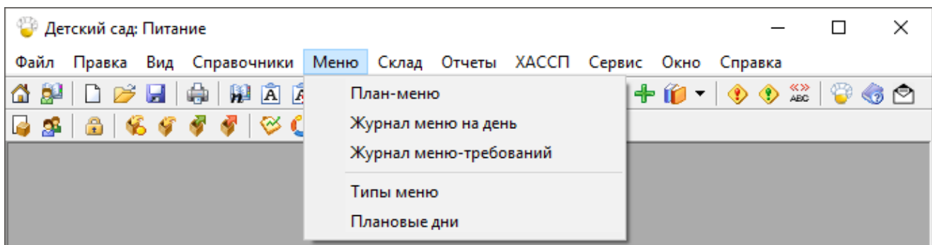
Меню «Меню»
