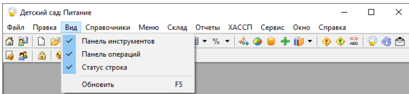
Меню «Вид»
