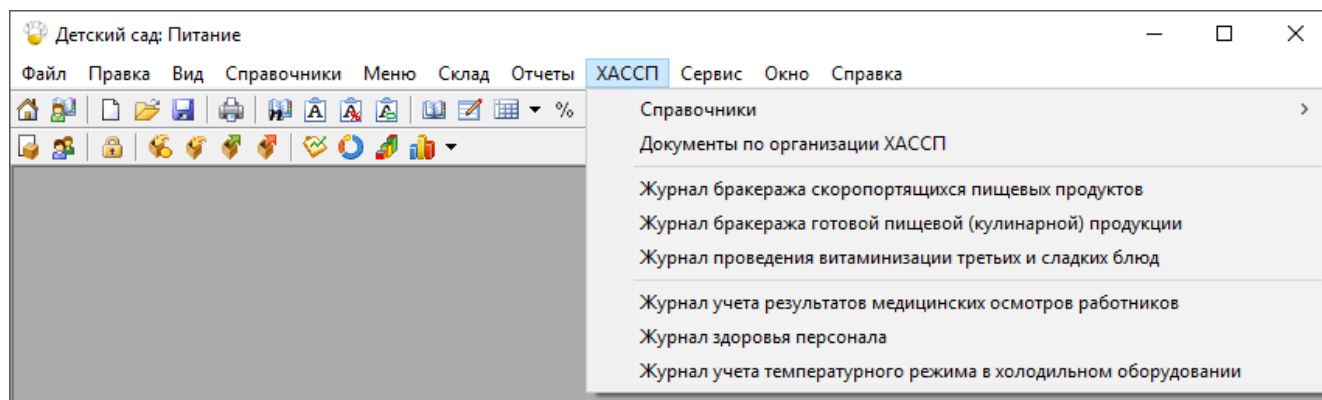
Меню «ХАССП»
