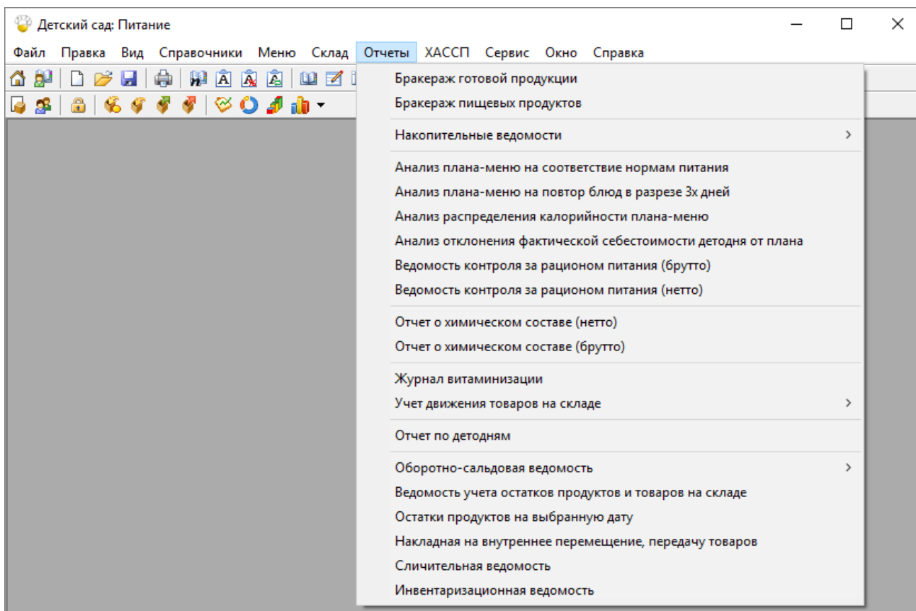
Меню «Отчеты»
