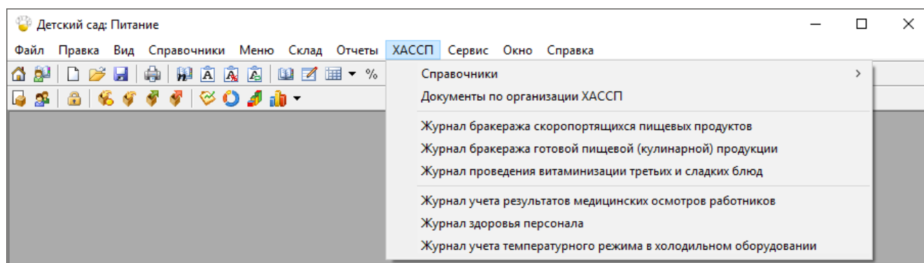
Меню «ХАССП»
