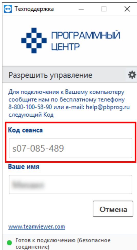
Код сеанса
