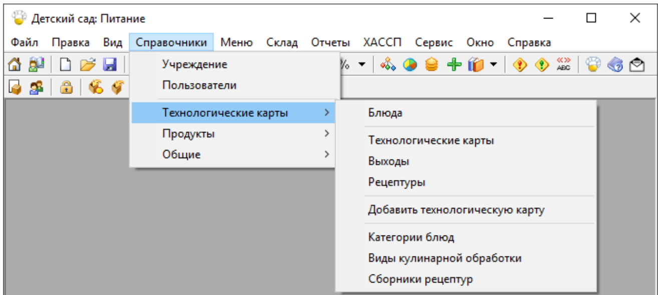
Меню «Справочники»
