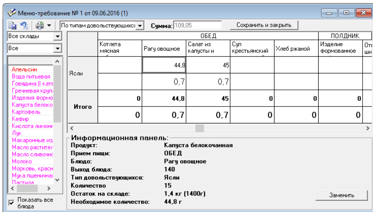
Окно «Меню-требования»
