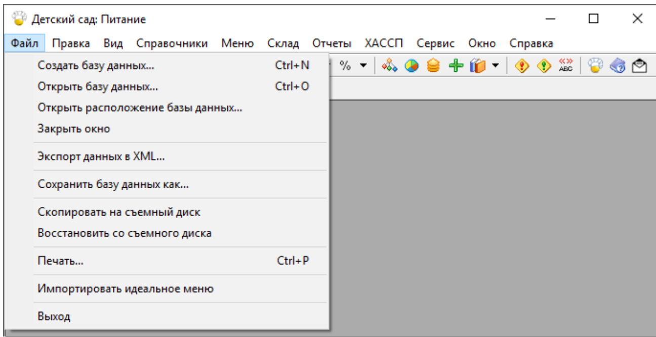
Меню «Файл»
