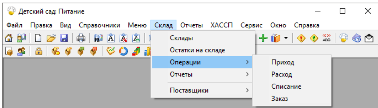
Меню «Склад»
