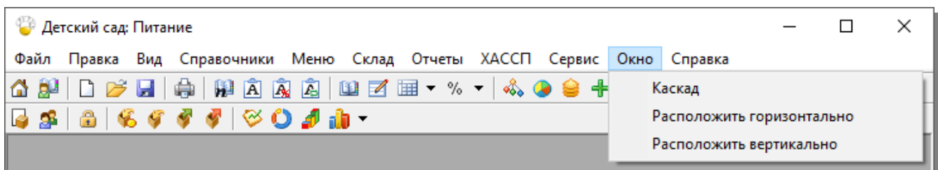
Меню «Окно»
