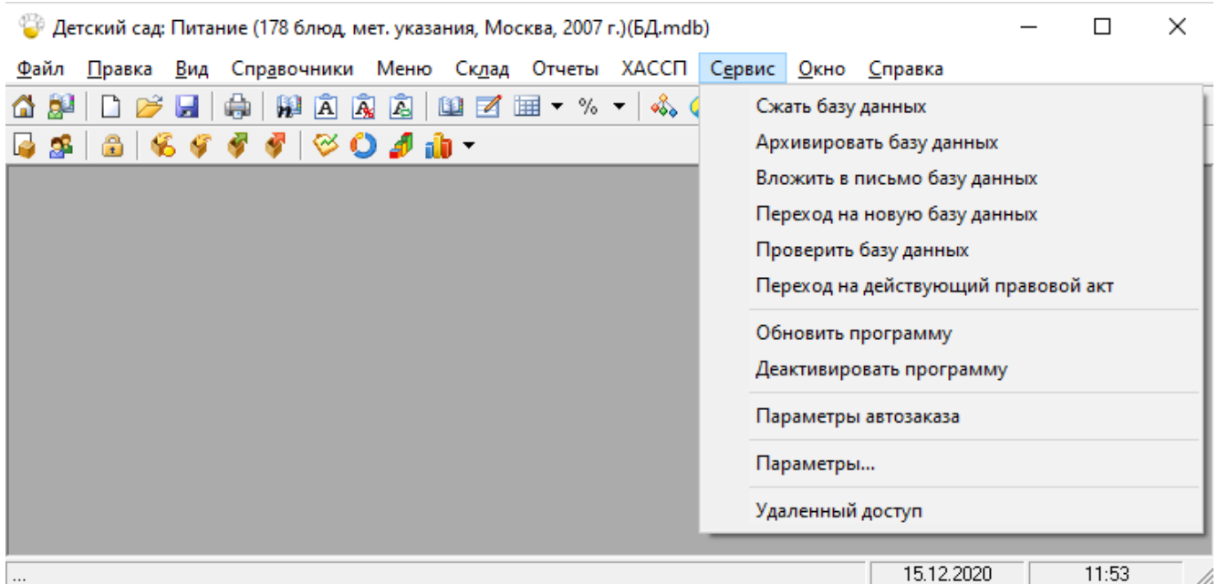
Меню «Сервис»
